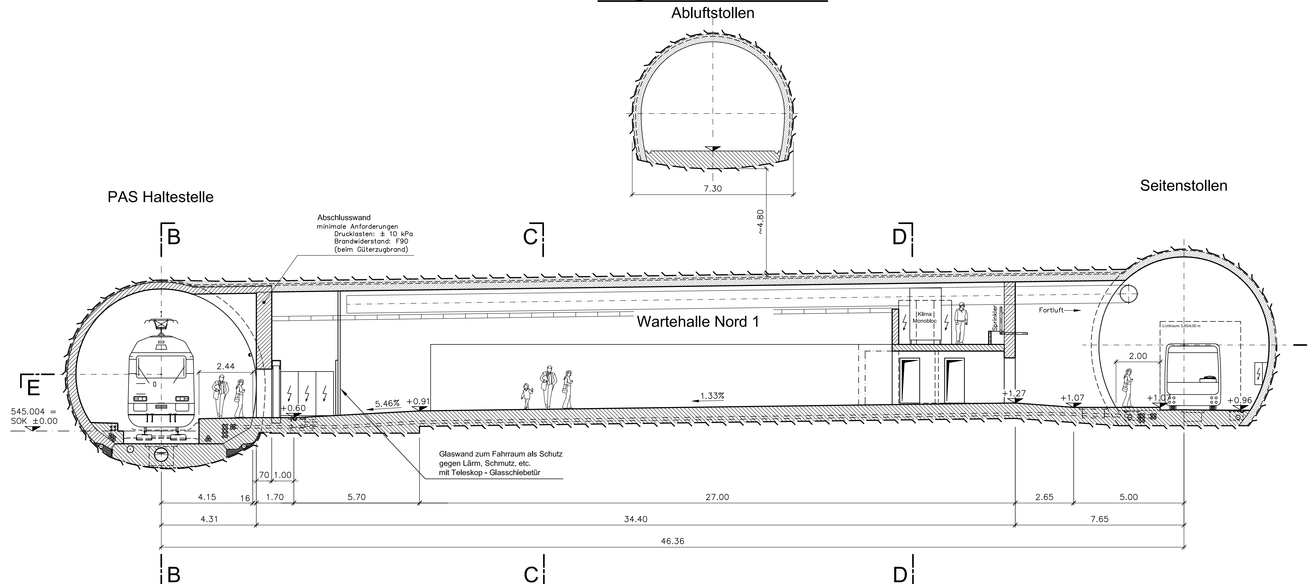
Längsschnitt A-A, 1:100
