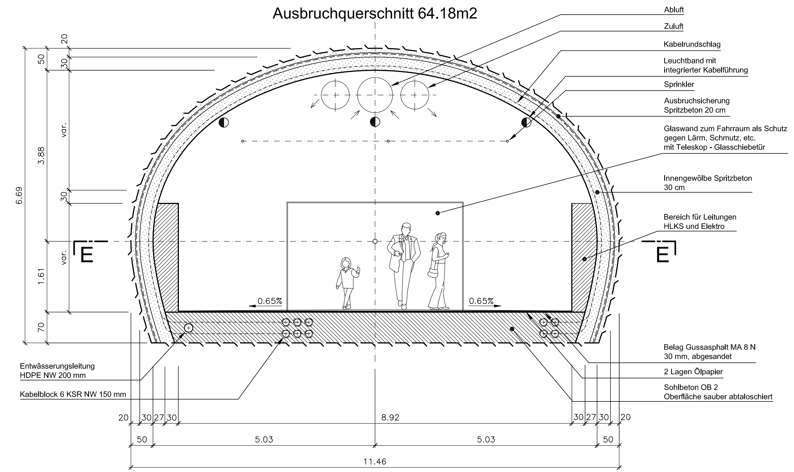
Schnitt C-C, 1:50
