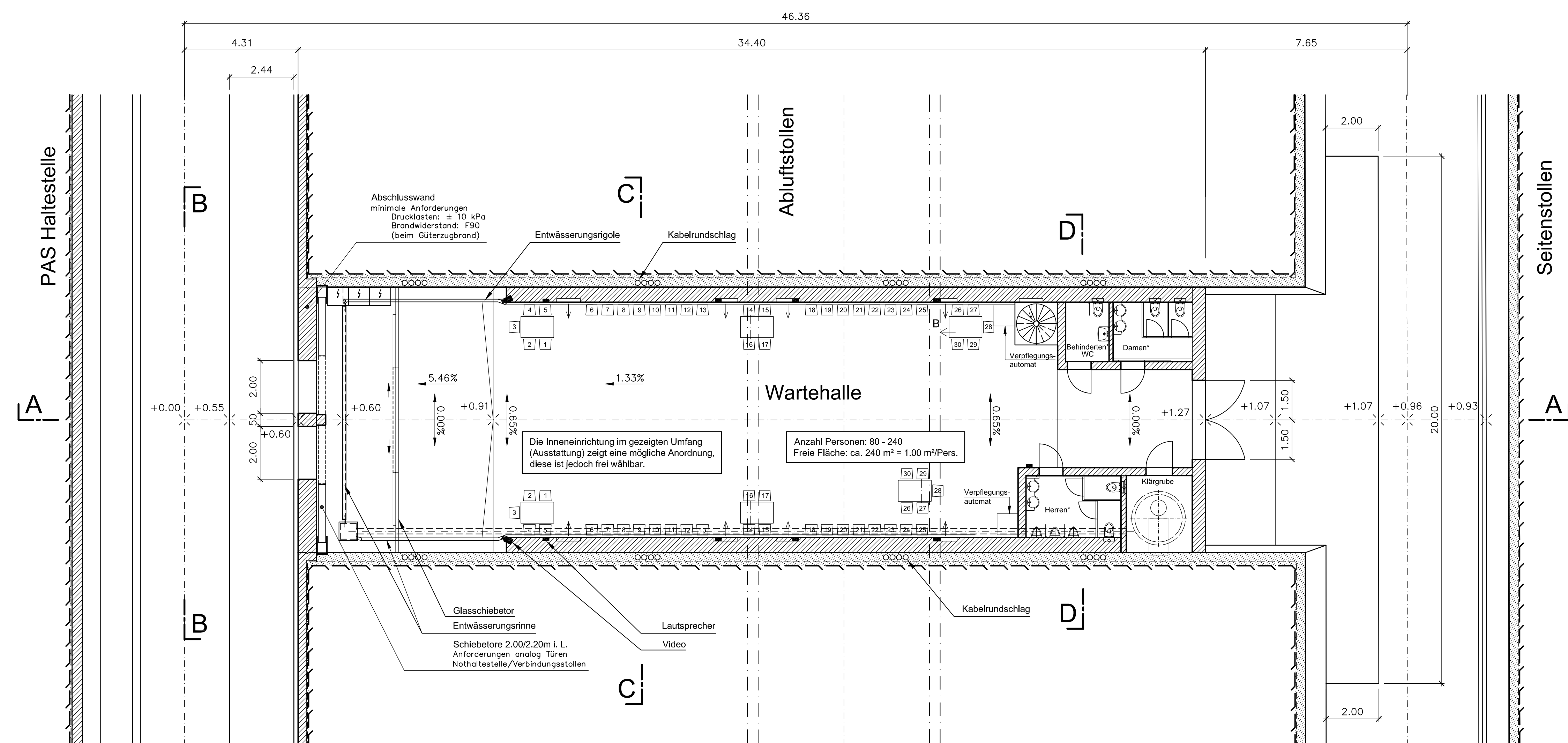
Grundriss E-E, 1:100
