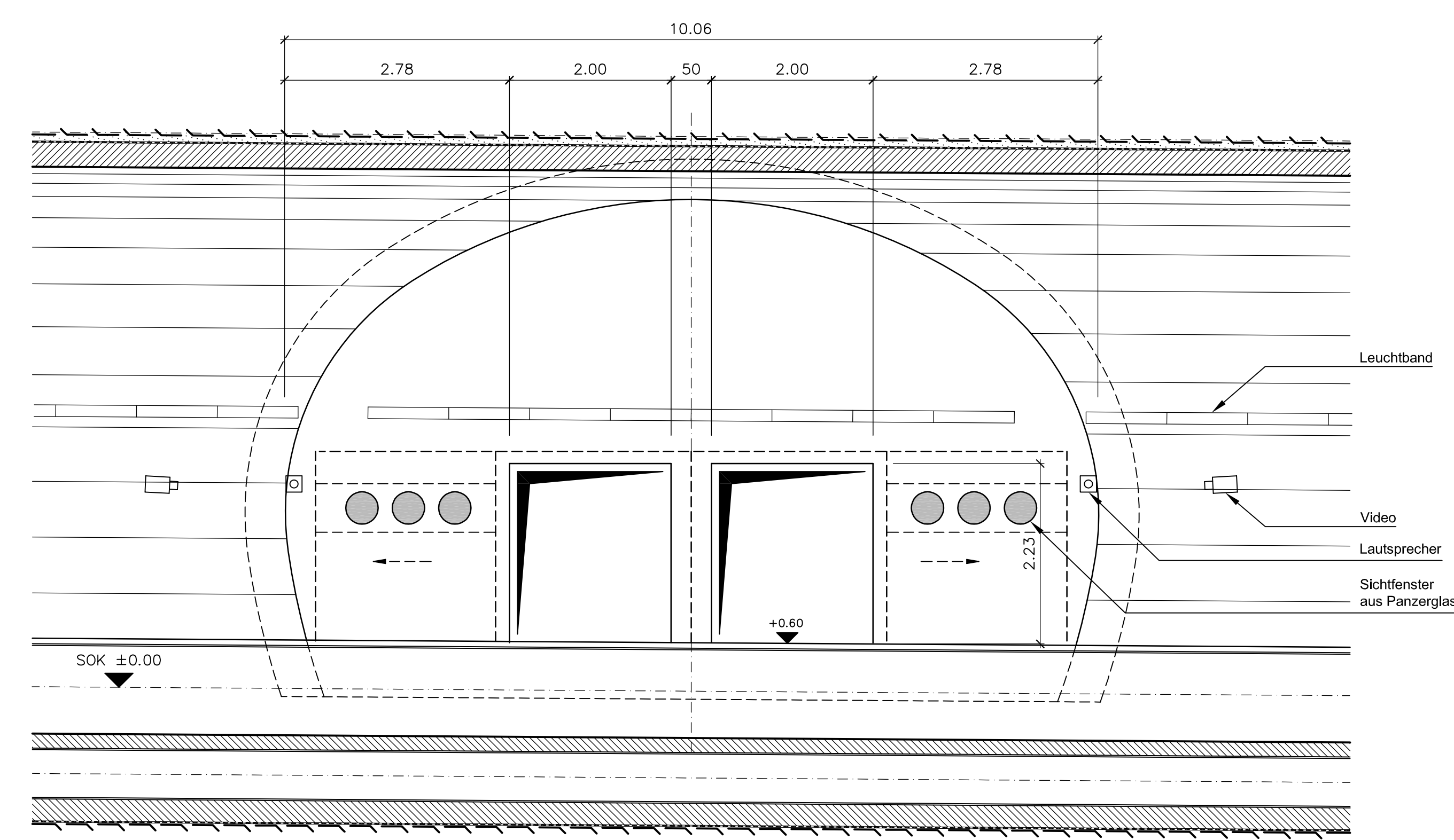
Schnitt B-B, 1:50
